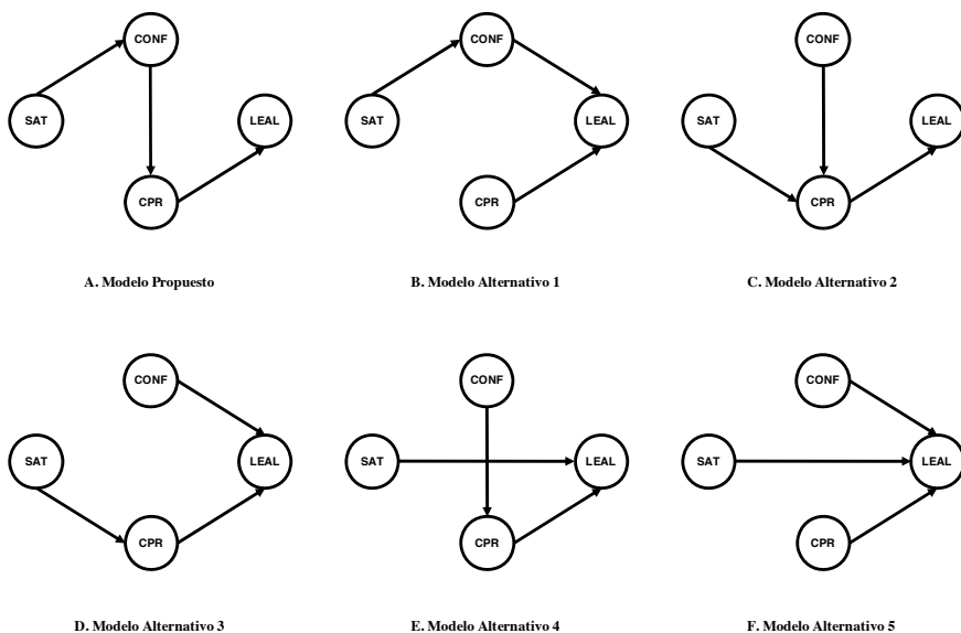
Figura 3 Modelo estructural causal y modelos rivales
